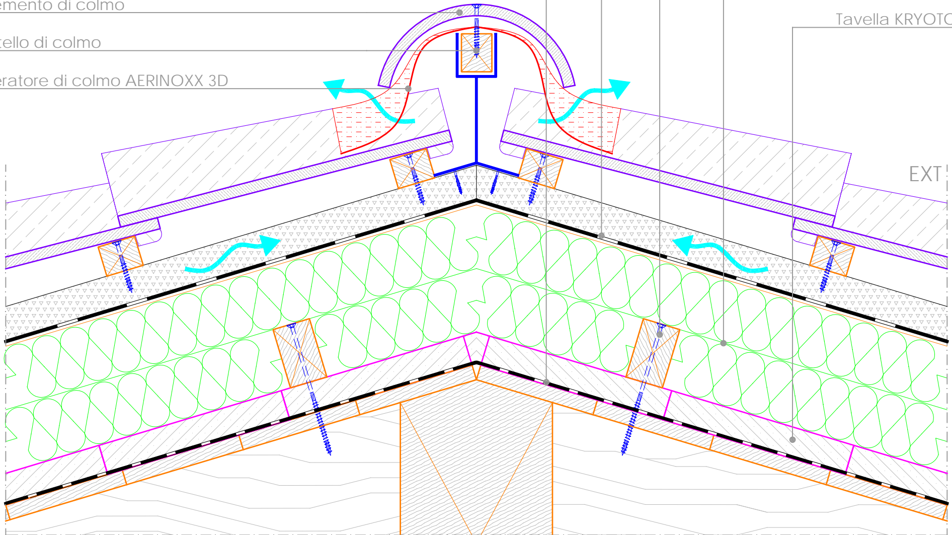
SEZIONE VERTICALE
