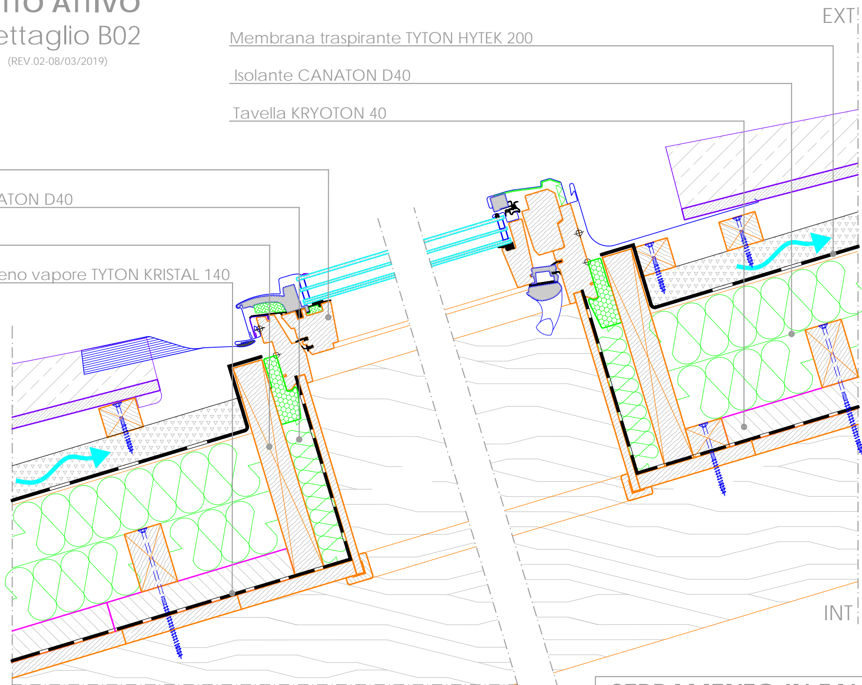
SEZIONE VERTICALE
