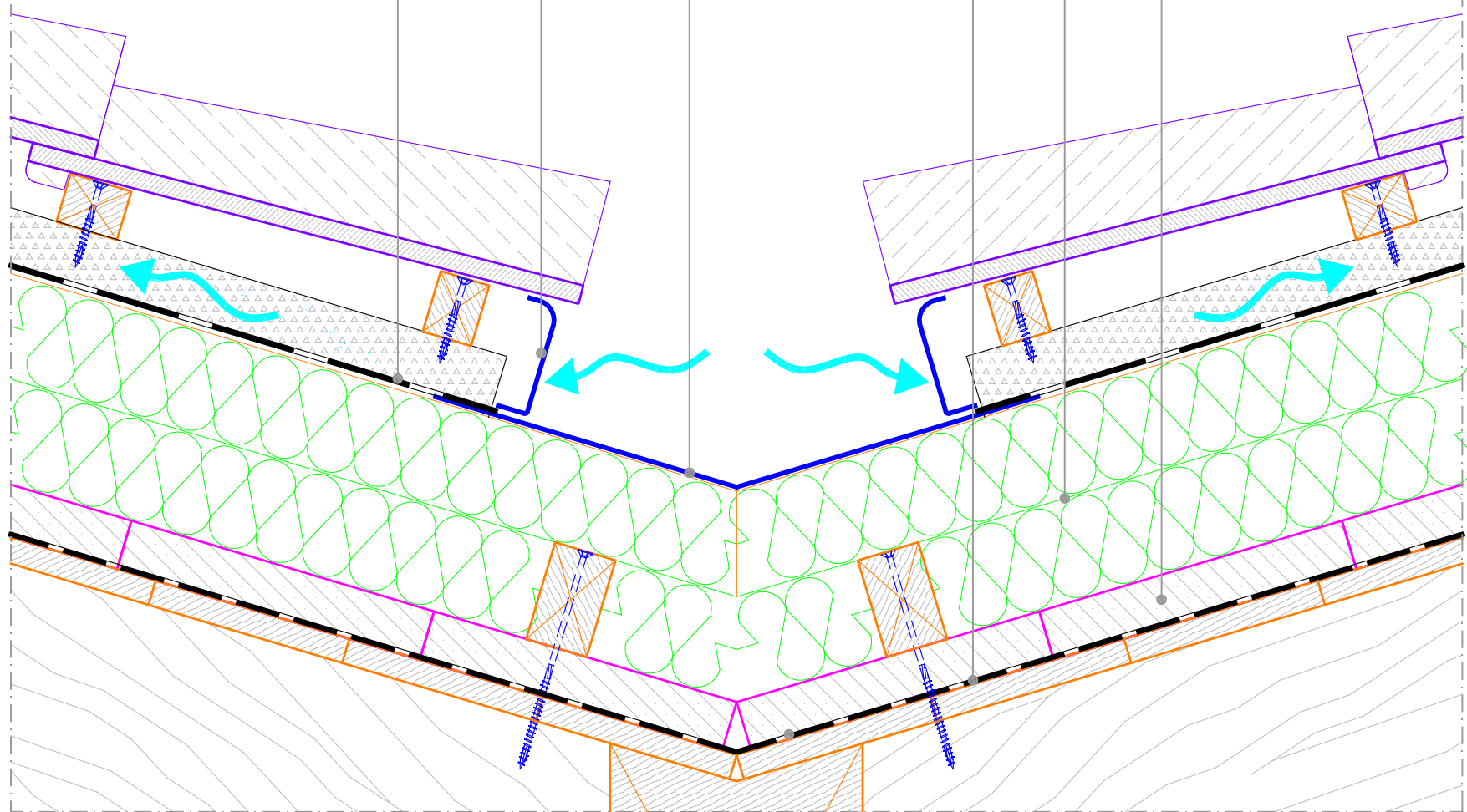
SEZIONE VERTICALE
