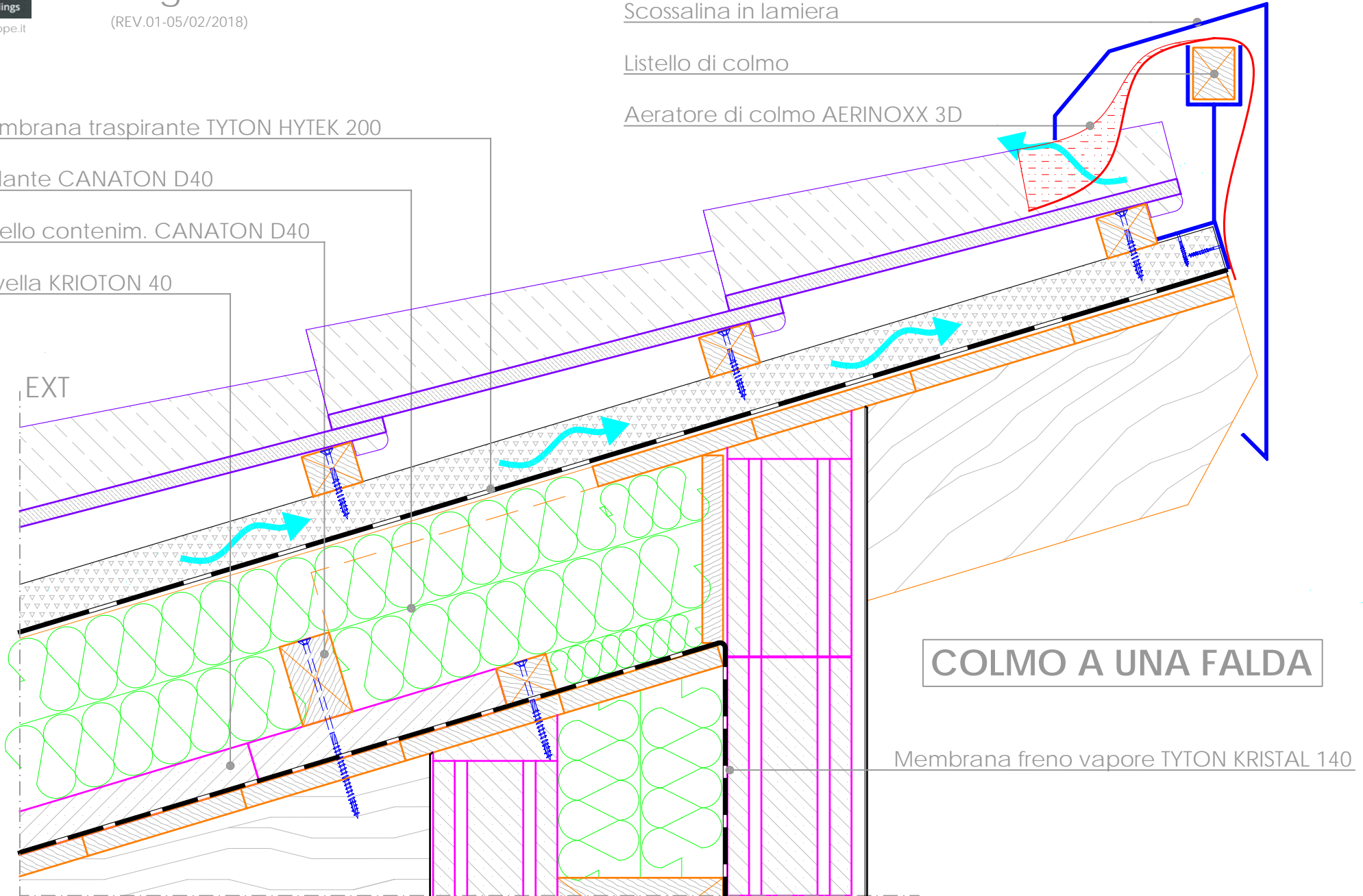
SEZIONE VERTICALE
