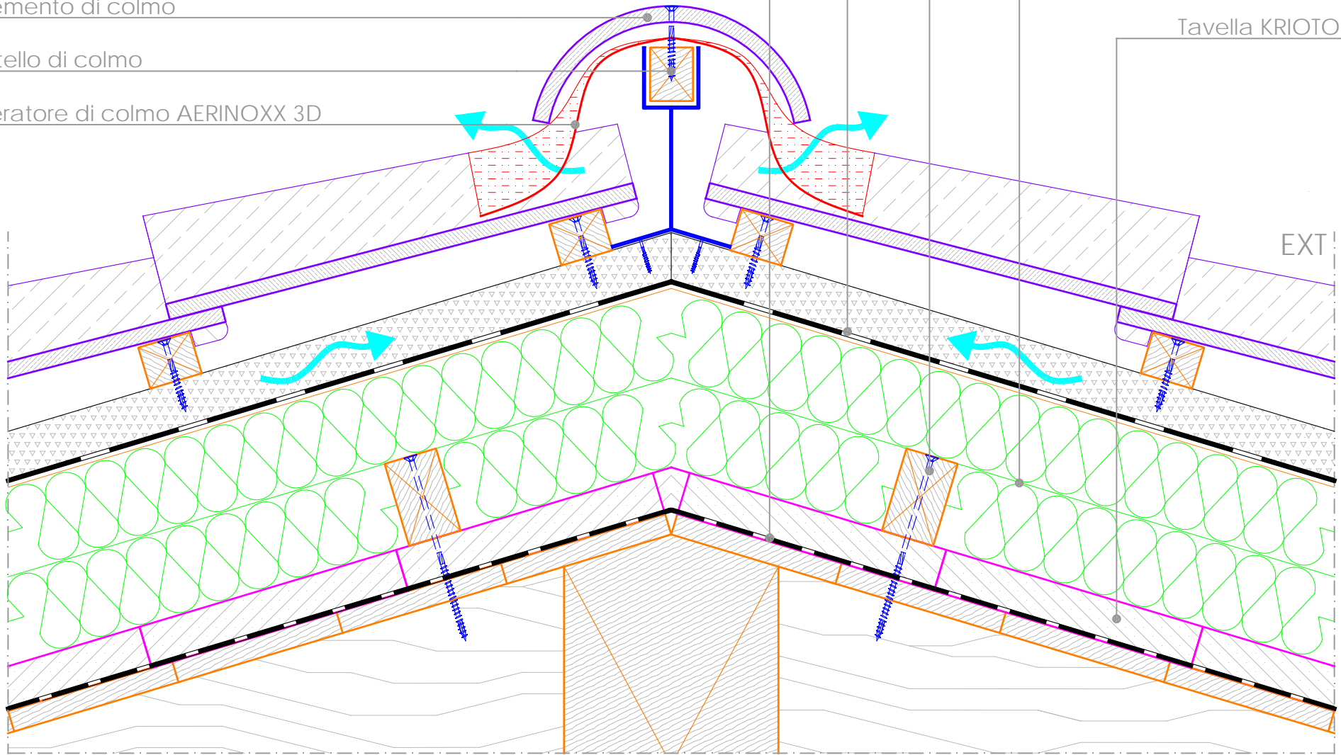
SEZIONE VERTICALE
