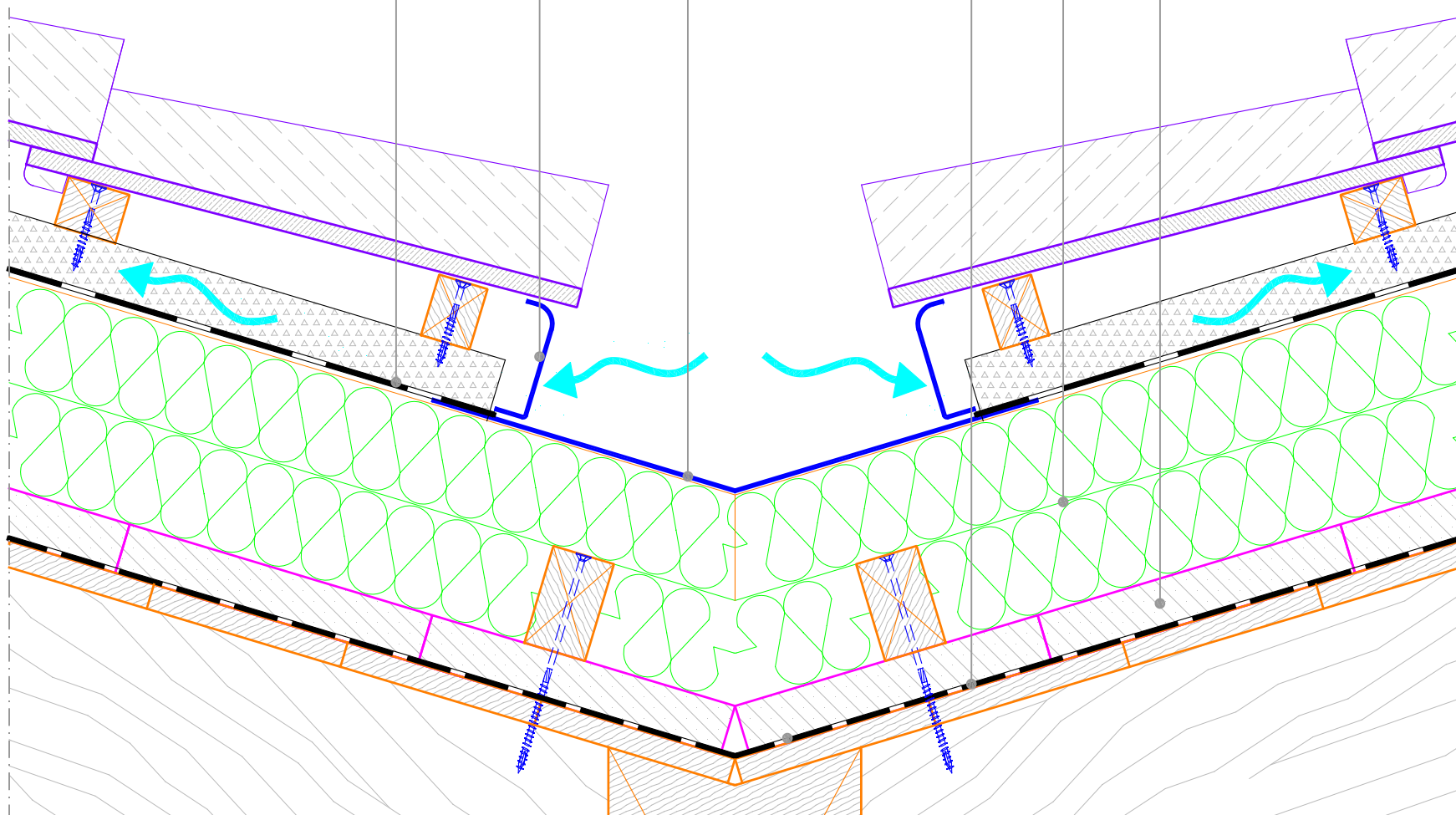
SEZIONE VERTICALE
