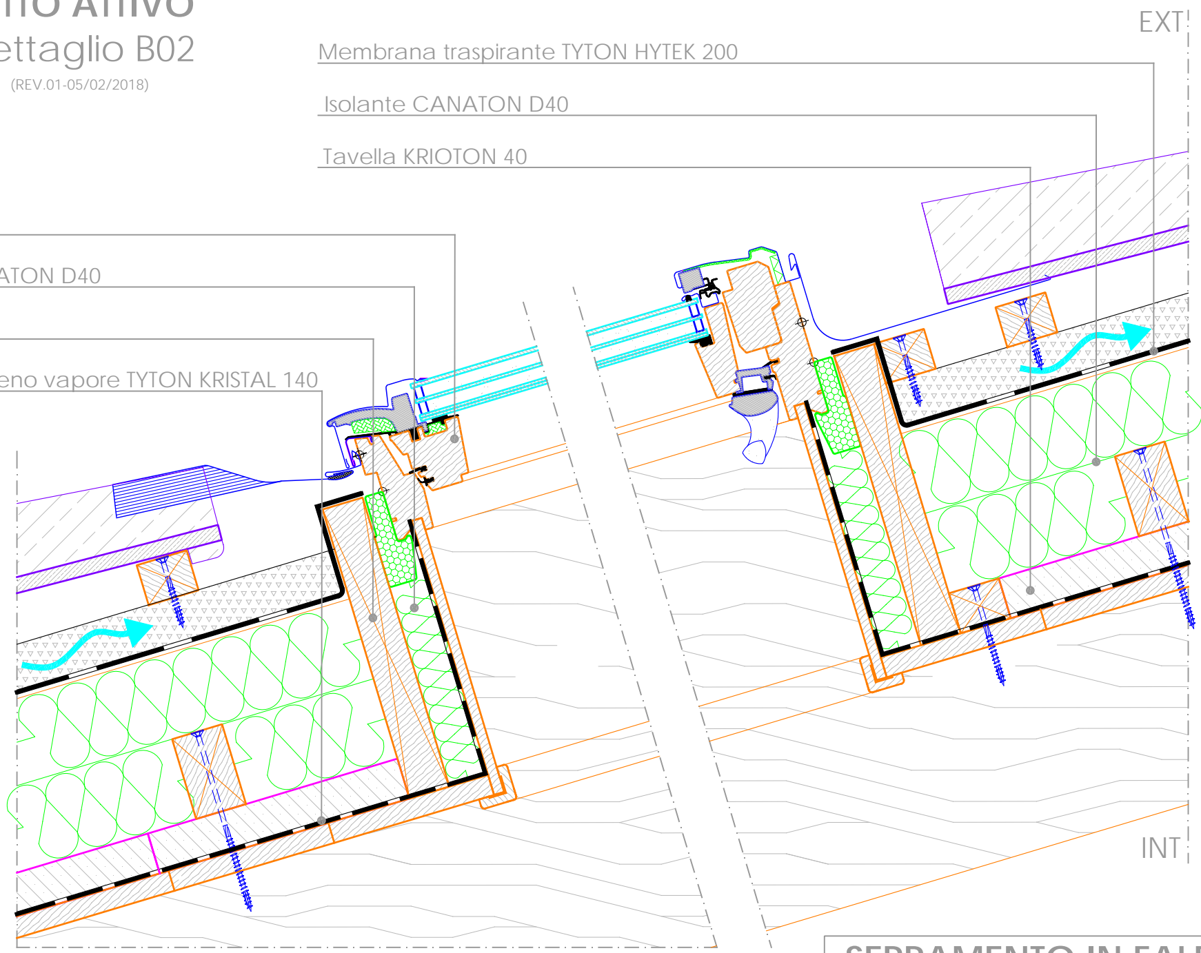
SEZIONE VERTICALE
