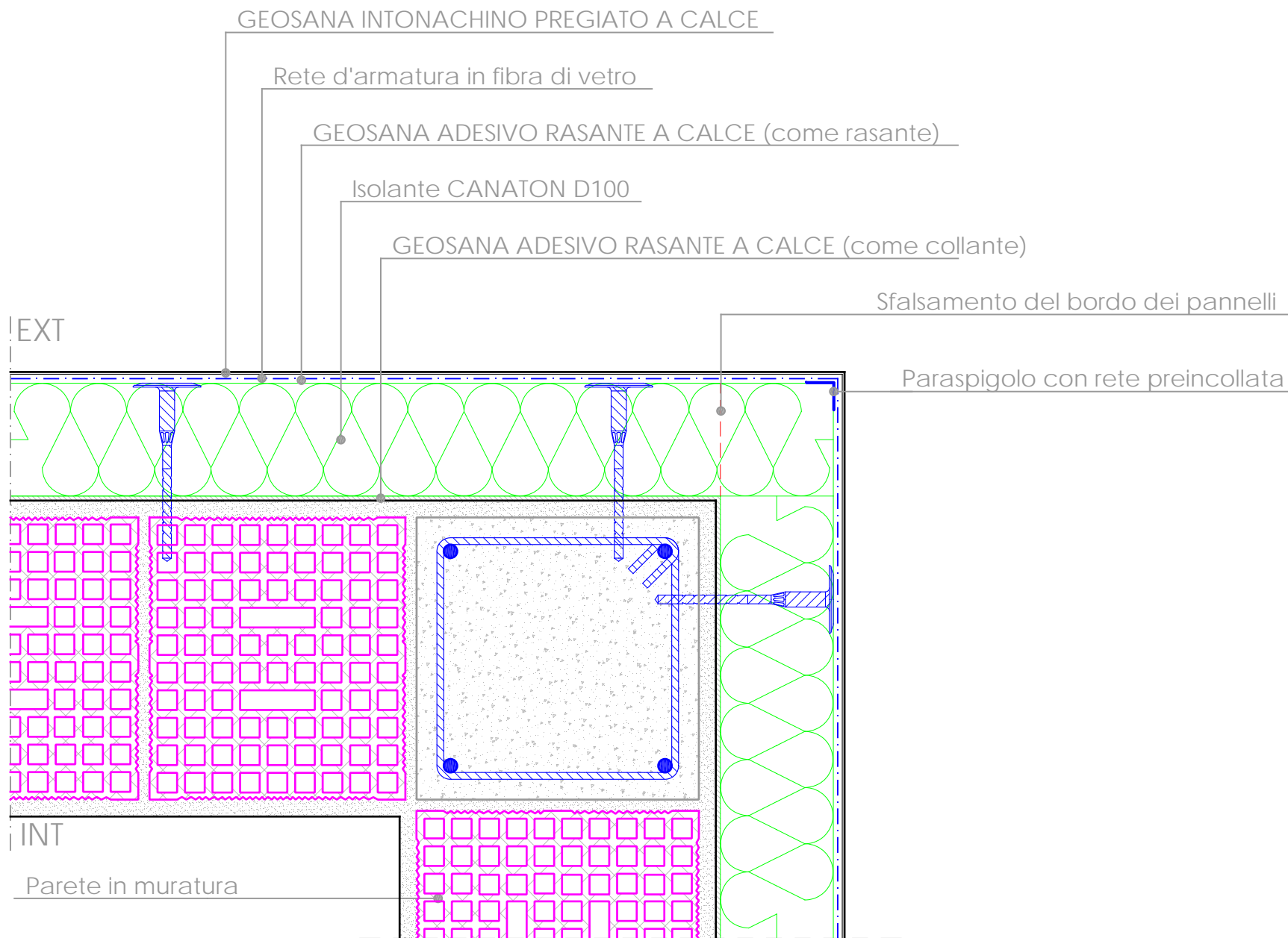
SEZIONE ORIZZONTALE
